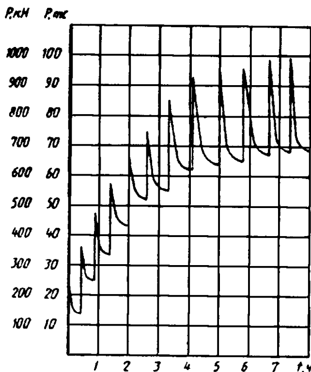
Рисунок 2 — График релаксации нагрузки за время испытания
