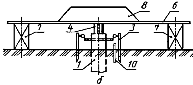
Установка с тарированным грузом
