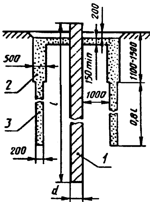
1 - испытываемая свая; 2 - траншея; 3 - дренажная скважина
