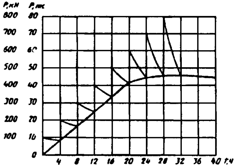
Рисунок 1 — График изменения нагрузки P во времени t
